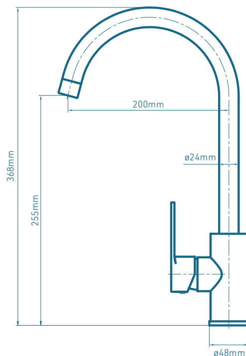
Desenho técnico (mm)
