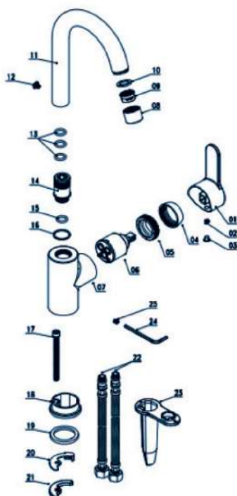
Desenho técnico
